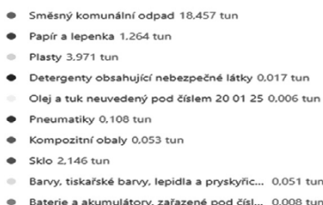
Sumarizační graf
